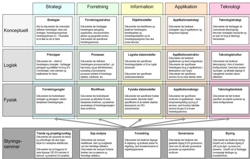
Figur 3: OIO's arkitekturrammeværk
